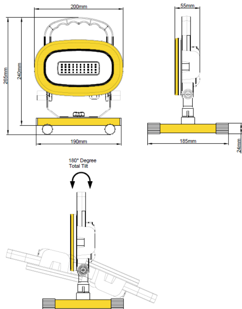
KSR5430 - Dimensions
