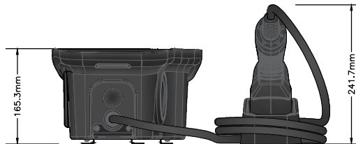
BOTTOM
